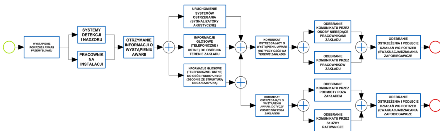
Rysunek: Schemat ostrzegania, alarmowania o zagrożeniu na terenie RLP Oddział w Sosnowcu oraz powiadamiania PSP
